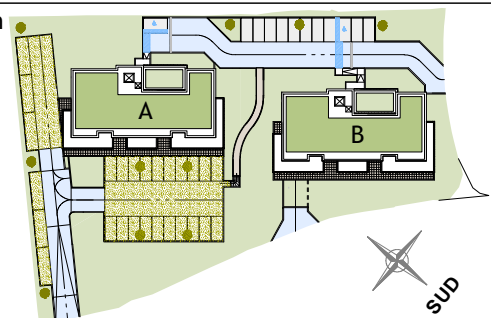
Bâtiment A - Appartement T3 - R+1 ou R+2
